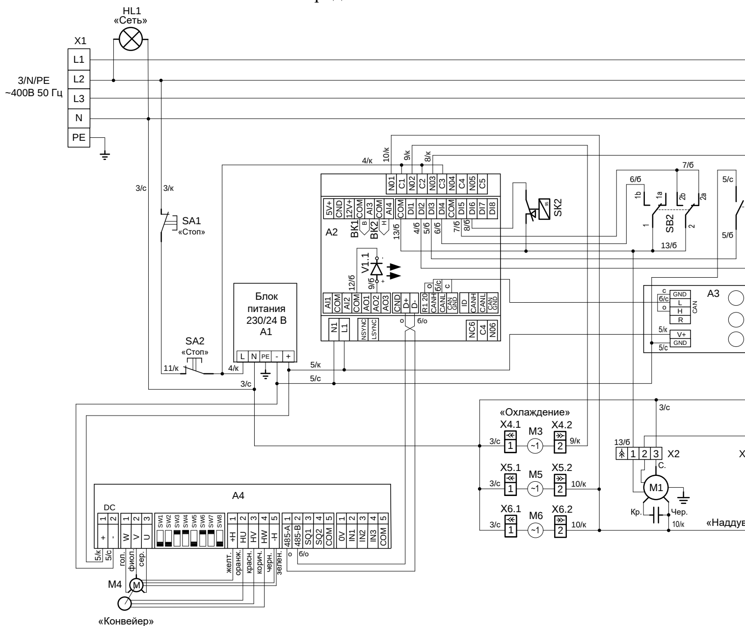
Рис. 16 - Схема электрическая принципиальная ПЭК-400 и ПЭК-400 с дверцей
