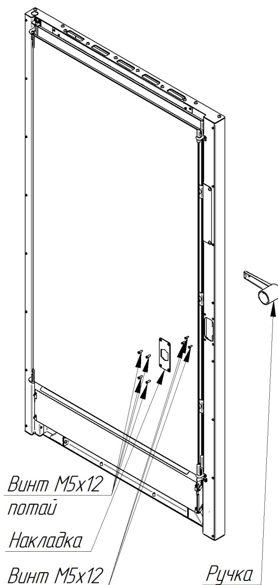
Рис. 16. Ремонт замкового устройства
