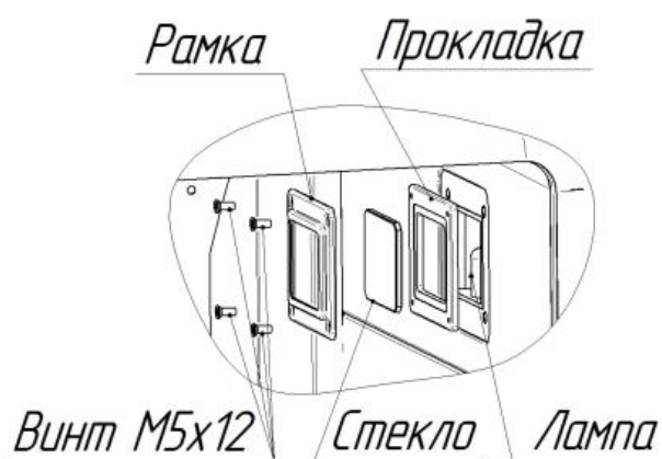
Рис. 18. Замена лампы освещения и прокладки
