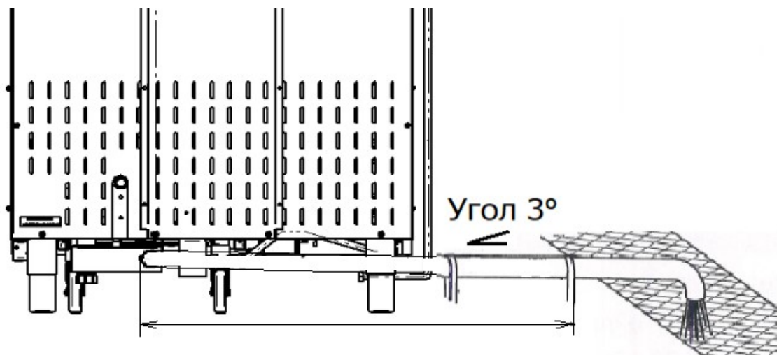
Рис. 8 Подключение пароконвектомата к канализации – слив в трап.
