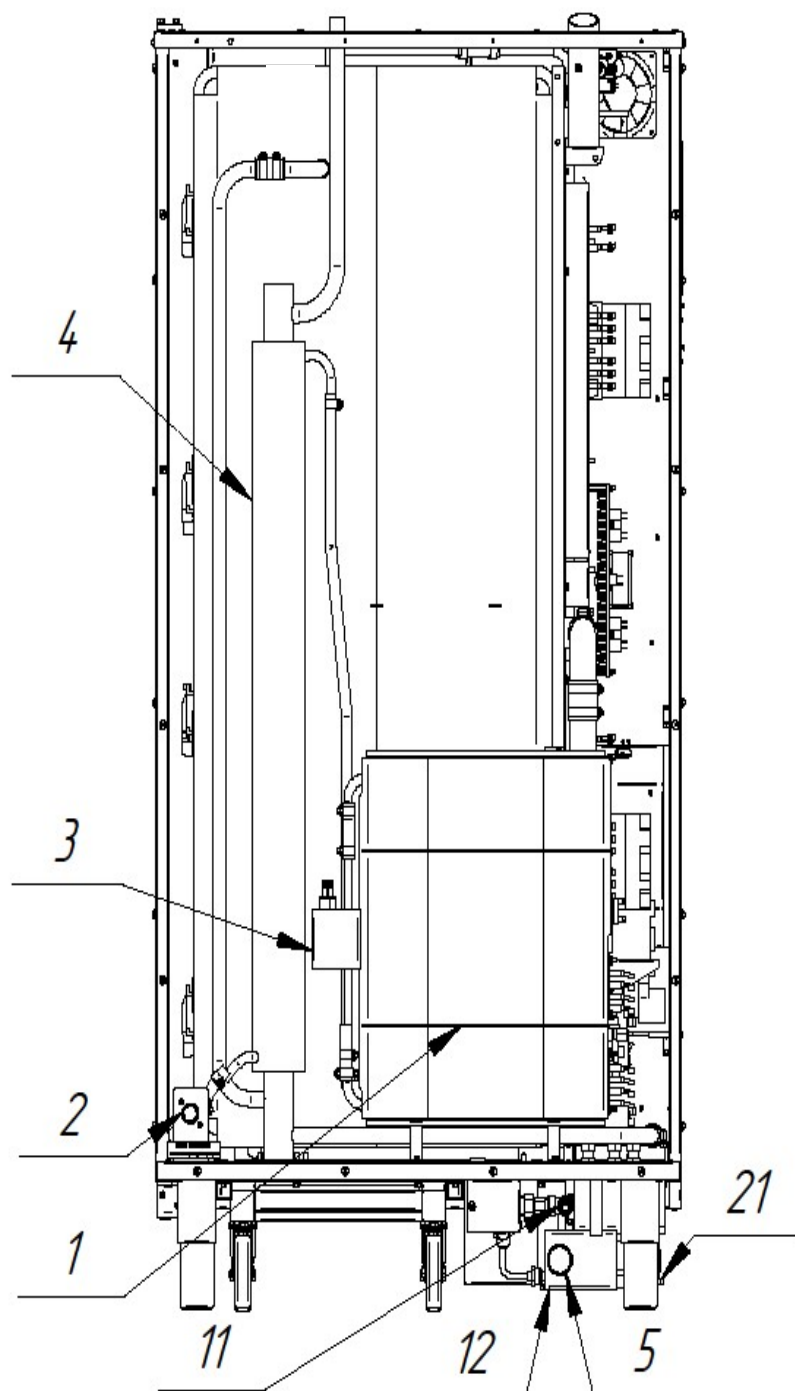
Рис.2а. Система водоснабжения, водоотведения и автоматической мойки (вид сзади)
