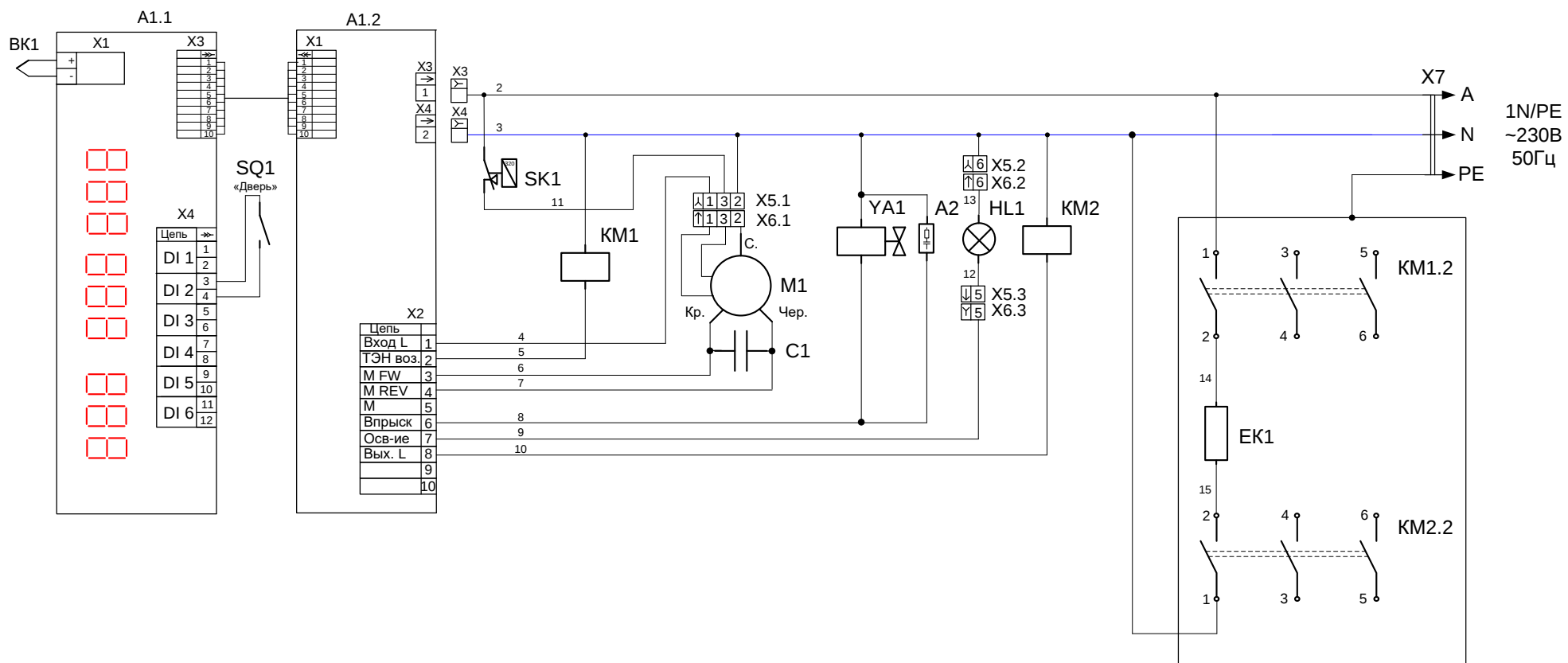
СХЕМА ЭЛЕКТРИЧЕСКАЯ ПРИНЦИПИАЛЬНАЯ КПП-4П, КПП-4ПЭ и КПП-4-1/2П
