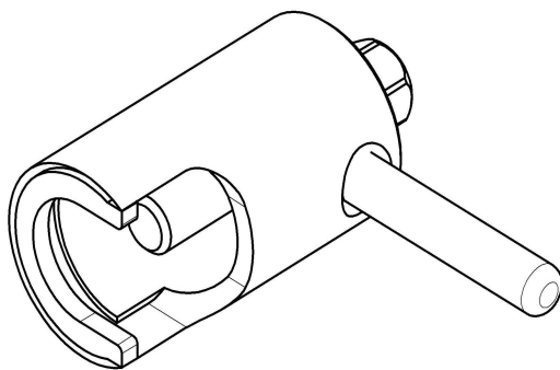
Рис. 17 Съемник крыльчатки(11000002907).
