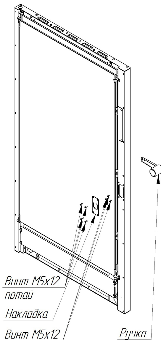
Рис. 20. Ремонт замкового устройства
