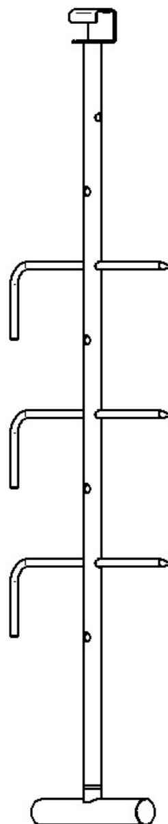
Рис.26. Общий вид спицы СТГ-20.
