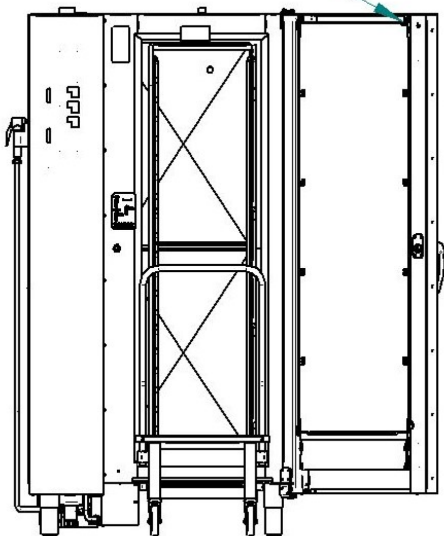
Рис. 15 Открывание внутреннего стекла.
