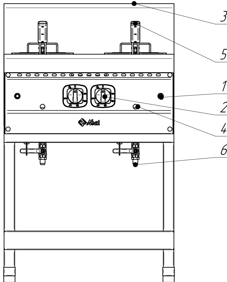
Рис. 1. Газовая фритюрница
